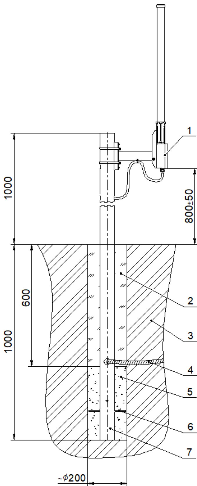
Рисунок 2.2 – Вариант установки извещателя на круглую опору в грунте.
