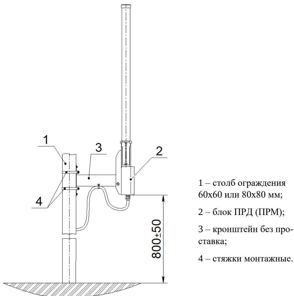
Рисунок 2.3 – Вариант установки извещателя на квадратный столб ограждения
